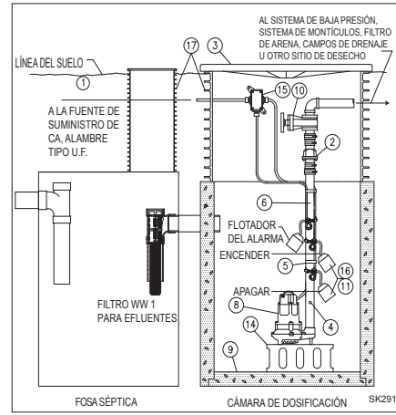
INSTALACIÓN TÍPICA PARA EFLUENTES
