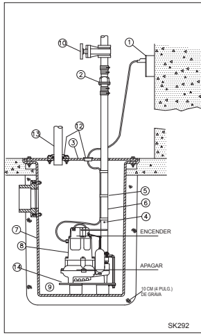
INSTALACIÓN TÍPICA PARA ACHIQUE
