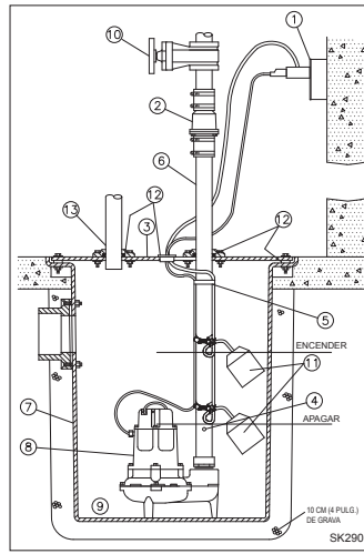
INSTALACIÓN TÍPICA PARA AGUAS CLOACALES
