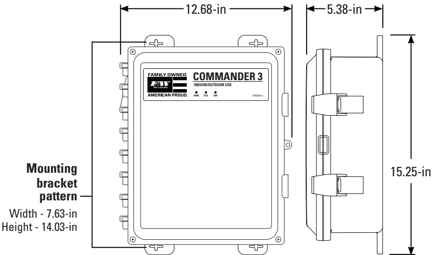
CMDR 2 & CMDR 3
